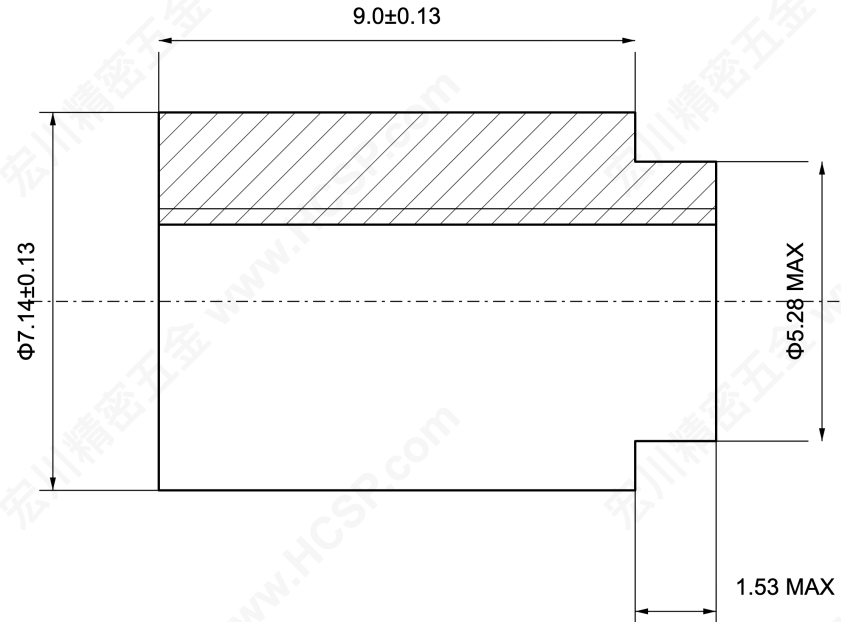
半剖视图 / HALF SECTION
