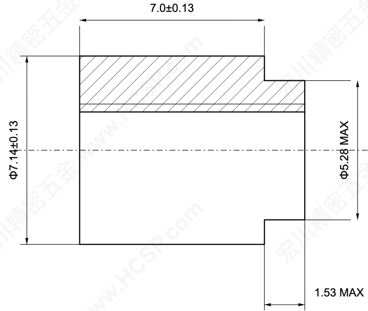
半剖视图 / HALF SECTION
