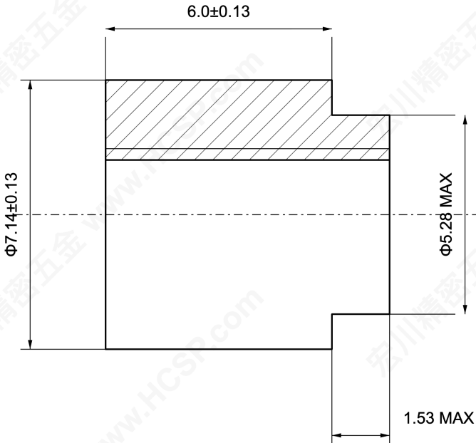
半剖视图 / HALF SECTION
