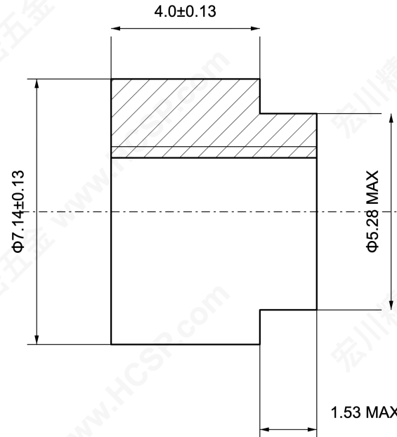
半剖视图 / HALF SECTION
