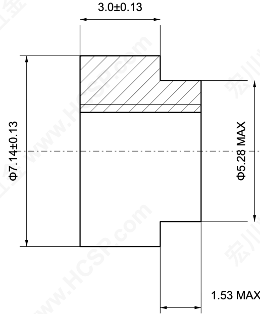
半剖视图 / HALF SECTION
