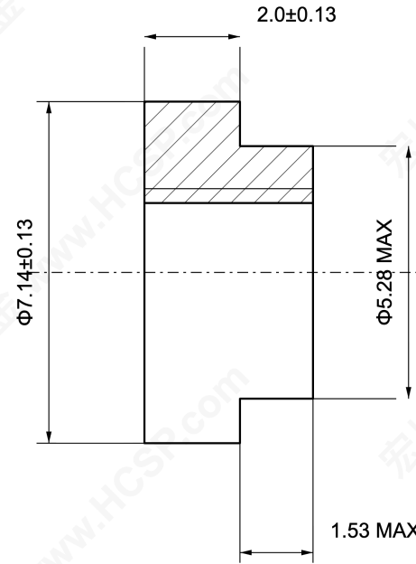
半剖视图 / HALF SECTION
