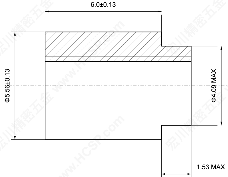
半剖视图 / HALF SECTION
