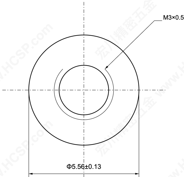
端视图 / END VIEW
