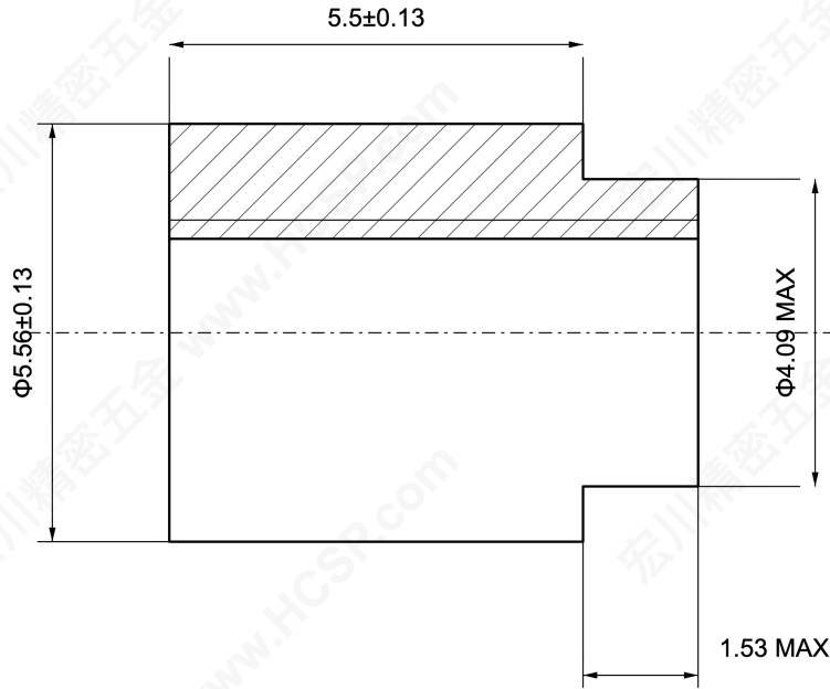
半剖视图 / HALF SECTION
