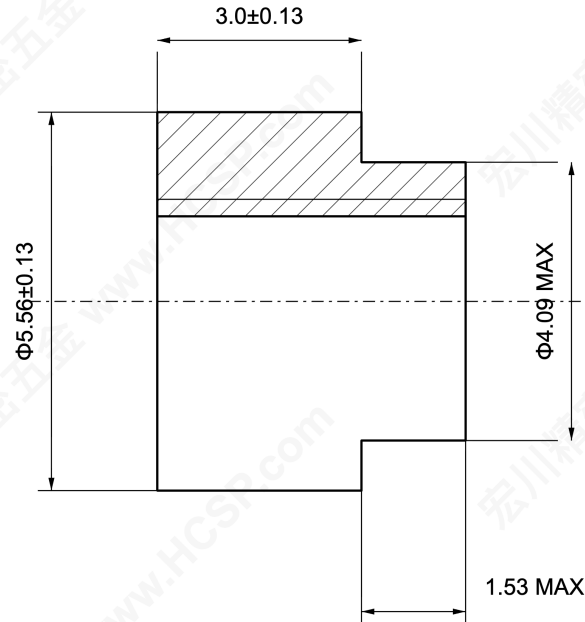
半剖视图 / HALF SECTION
