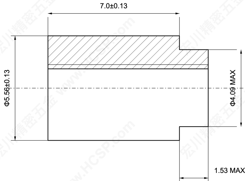
半剖视图 / HALF SECTION
