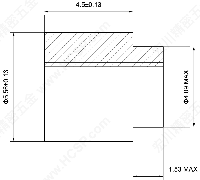
半剖视图 / HALF SECTION
