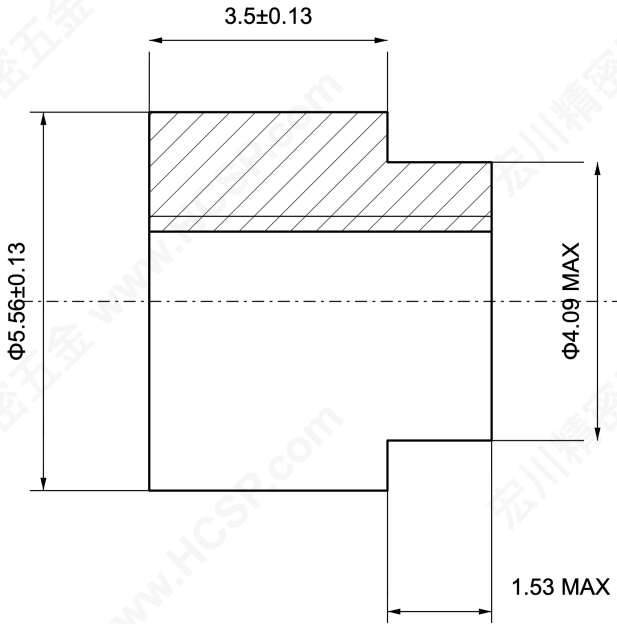
半剖视图 / HALF SECTION
