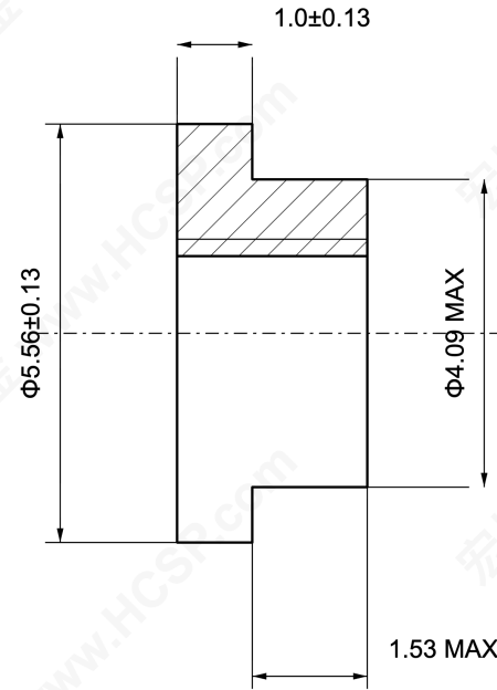
半剖视图 / HALF SECTION
