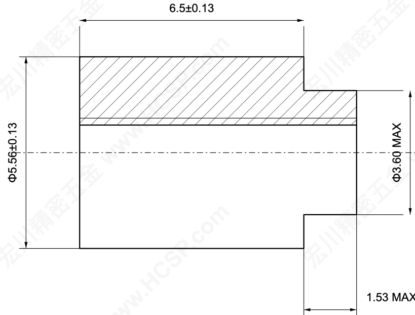
半剖视图 / HALF SECTION
