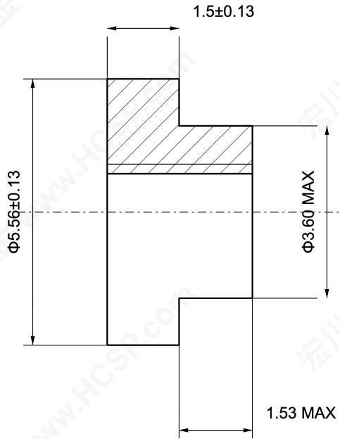
半剖视图 / HALF SECTION
