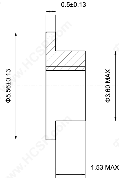
半剖视图 / HALF SECTION
