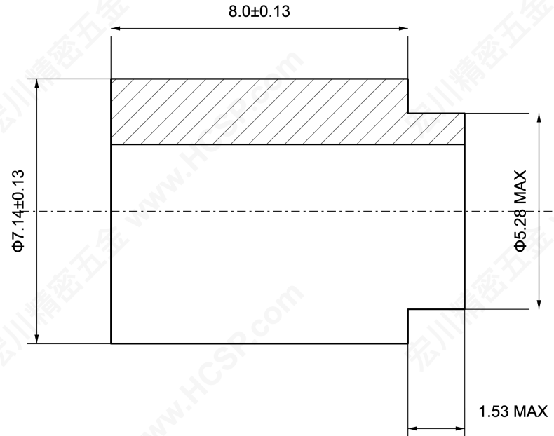
半剖视图 / HALF SECTION
