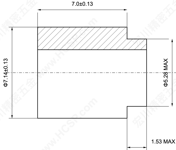
半剖视图 / HALF SECTION
