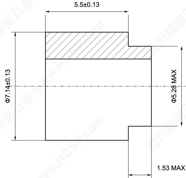
半剖视图 / HALF SECTION
