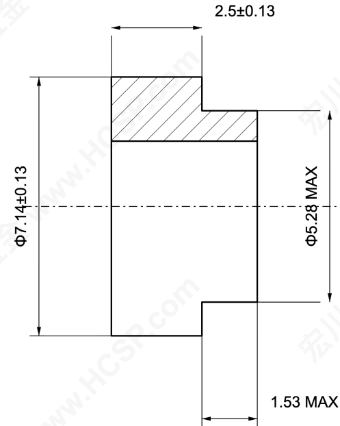
半剖视图 / HALF SECTION
