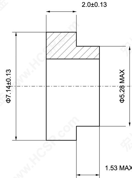
半剖视图 / HALF SECTION
