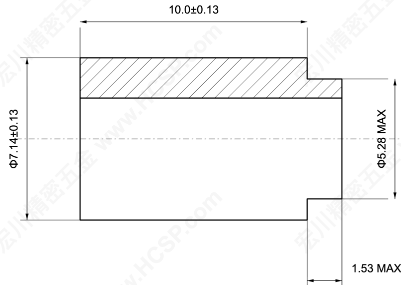
半剖视图 / HALF SECTION
