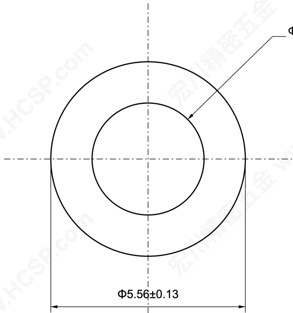
端视图 / END VIEW
