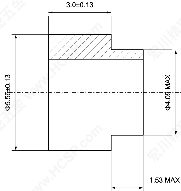
半剖视图 / HALF SECTION
