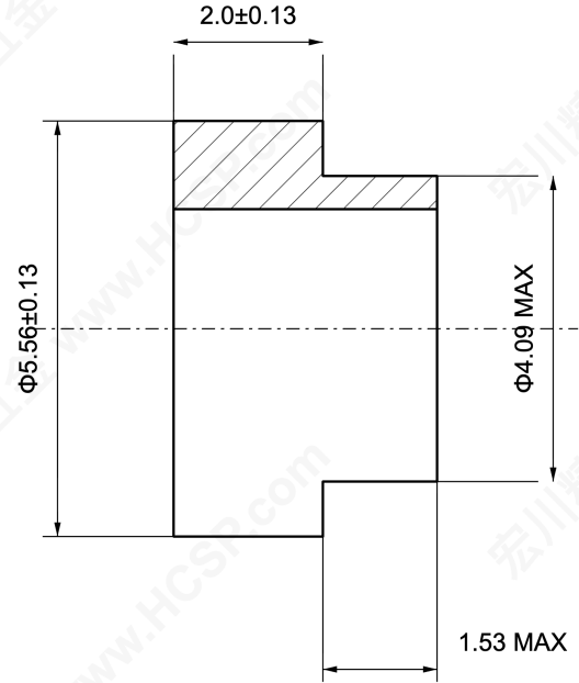
半剖视图 / HALF SECTION
